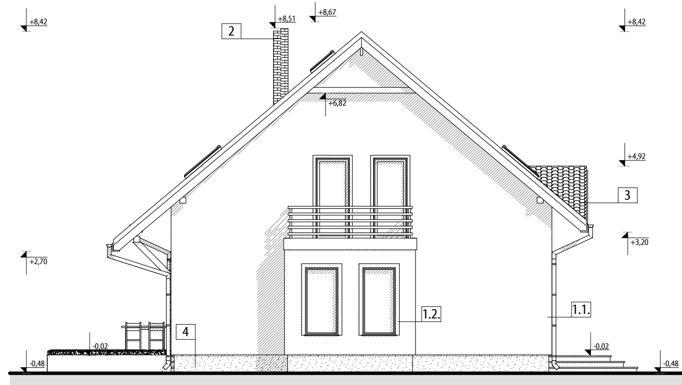
ELEWACJA POŁUDNIOWA- BOCZNA
