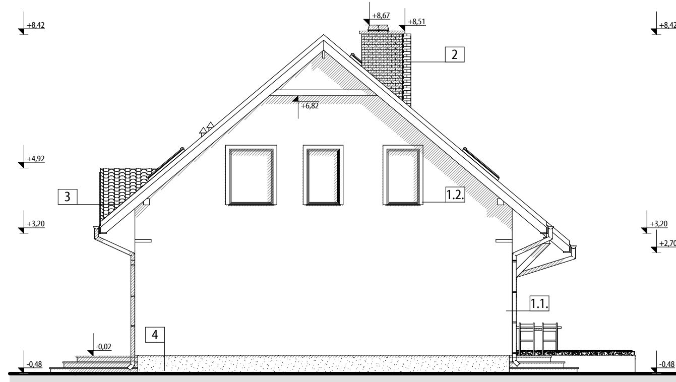
ELEWACJA PÓŁNOCNA- BOCZNA
