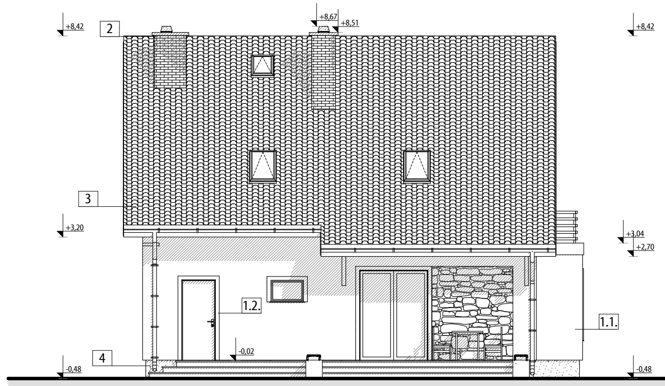
ELEWACJA ZACHODNIA- OGRODOWA
